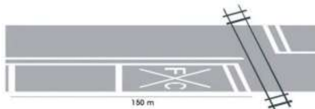
Marcas para el cruce del ferrocarril
